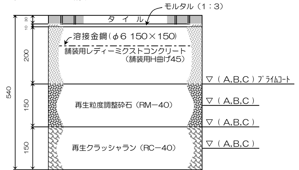
17. カラータイル舗装 54型
