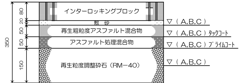
16. 歩道乗入舗装 35型 (インターロッキング)
