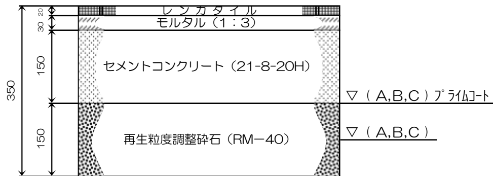
15. 歩道乗入舗装 35型 (レンガタイル)
