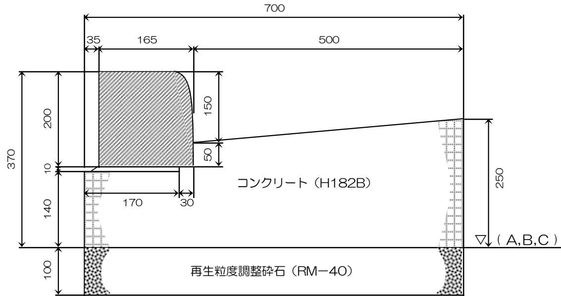
38. 街きょ
