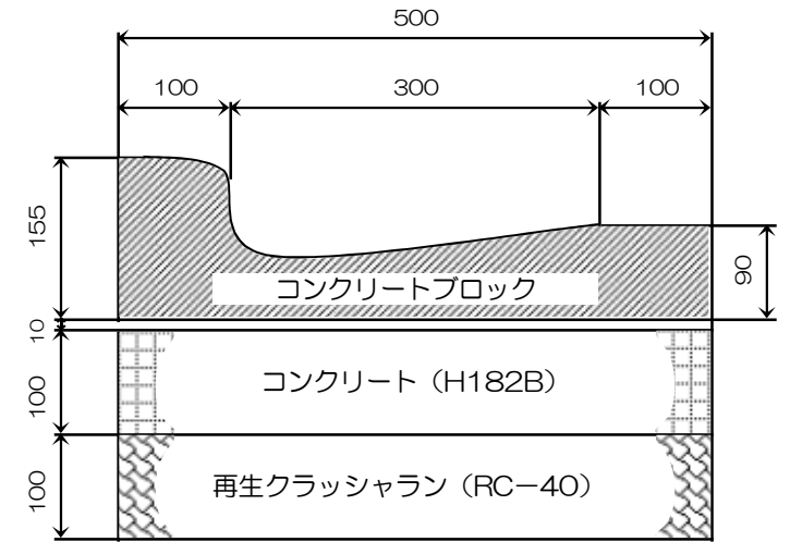
39. L形側溝
