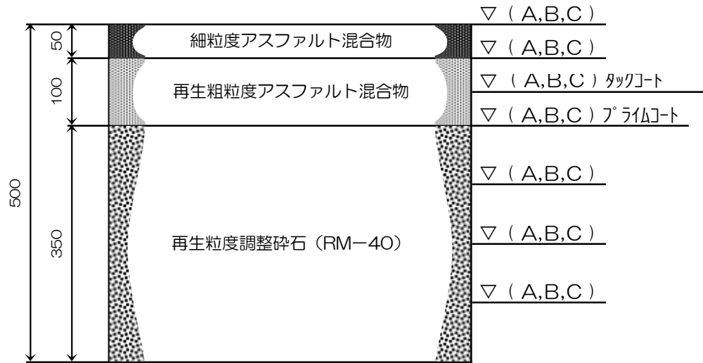
14. 歩道乗入舗装 50型 (アスコン)
